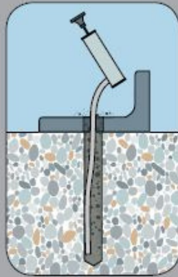
Očistiti rupu izduvavanjem
