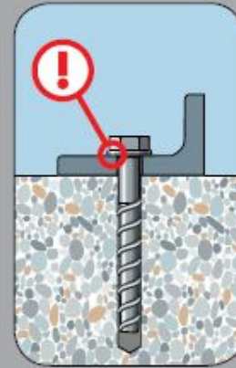
Montaža: Anker je montiran kada dobro nalegne na profil koji se pričvršćuje
