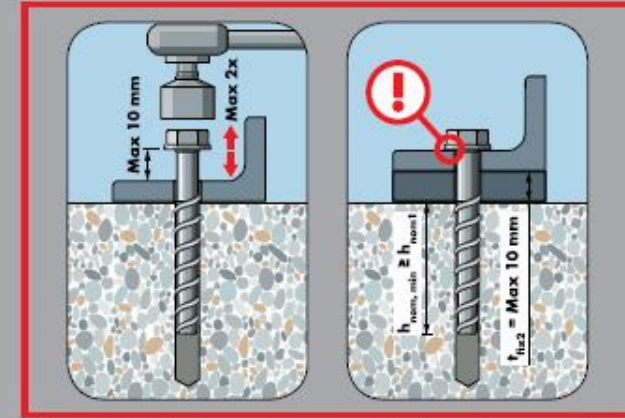
Najviše dva puta odvrnuti /zavrnuti anker prilikom podešavanja u ukupnoj dužini od 10mm
